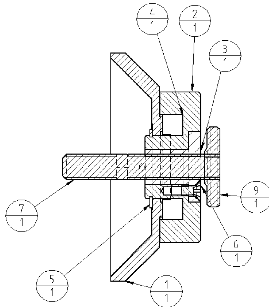
SCHNITT A-A
